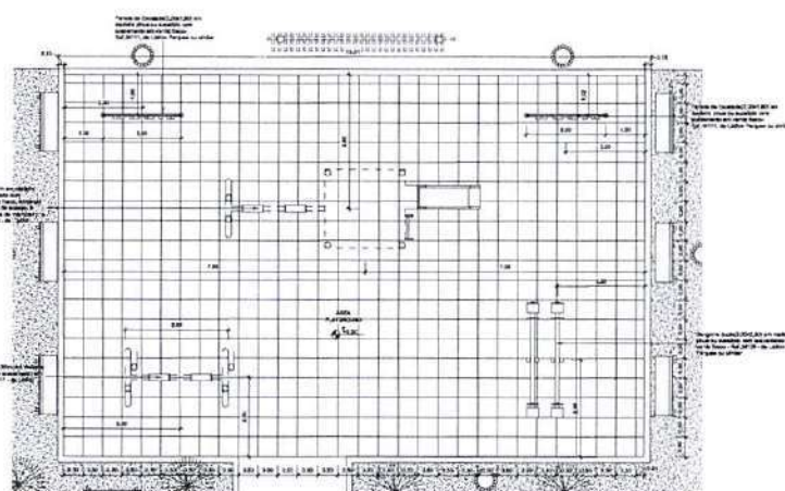
3 PLANTA BAIXA - Playground Executivo 1:50
