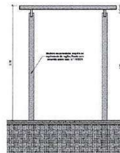
4 Corte 4 1:25
