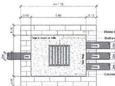
Planta Baixa - Caixa de Passagem Pluvial
