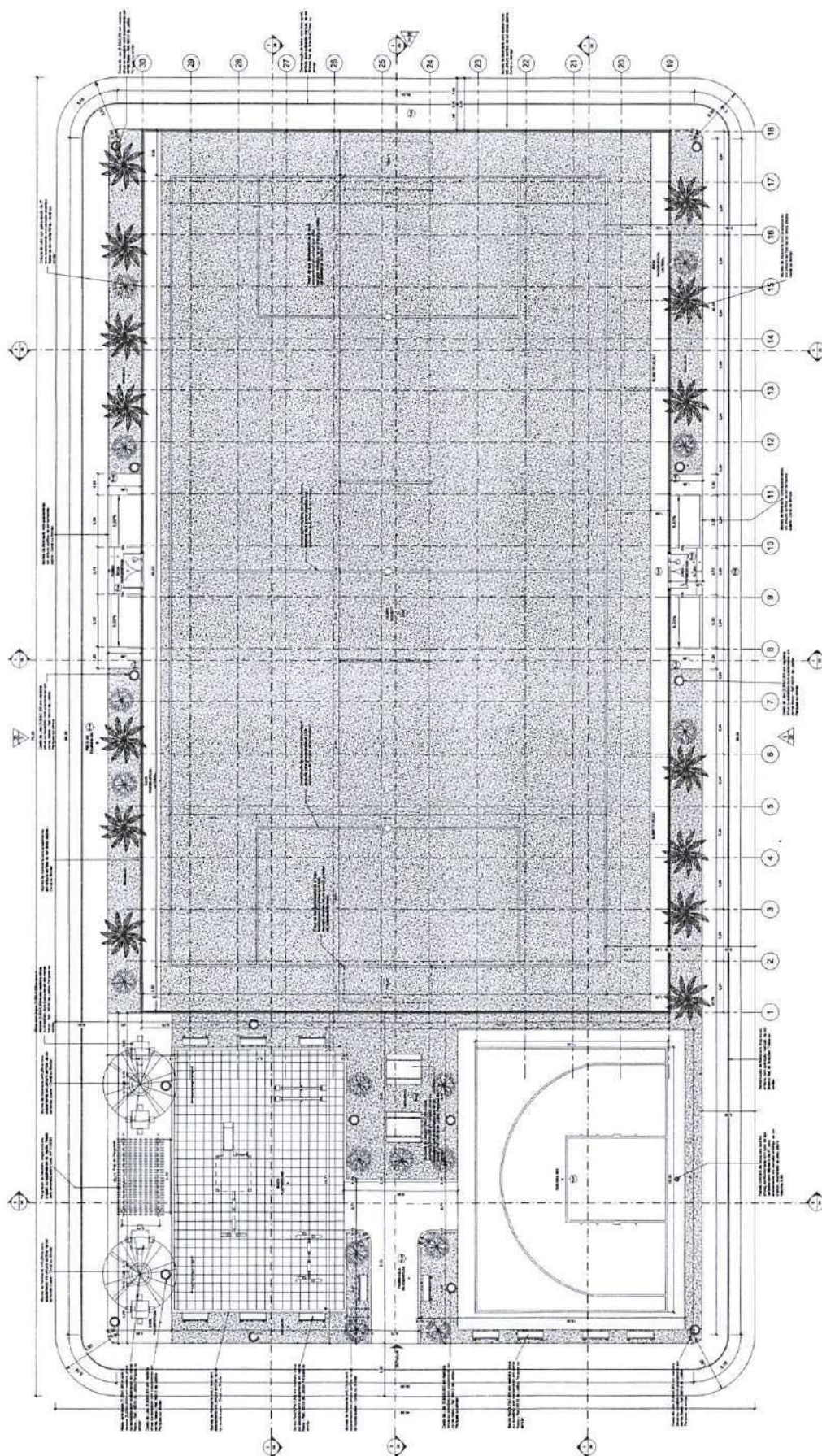
1 PLANTA BAIXA 1:75
