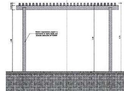
5 Corte 5 1:25
